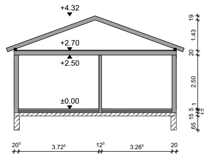
Schnitt A-A
